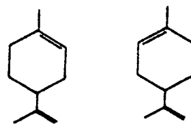
Limonene (Dipentene)
