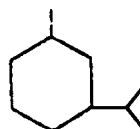
m-Menthane
